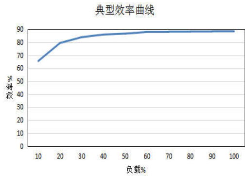
12V 输出典型效率曲线
