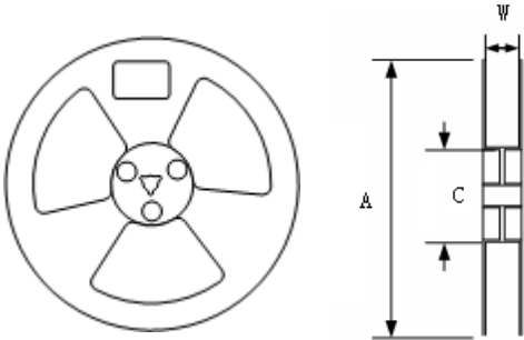
(2) 卷盘尺寸 Taping reel dimensions
