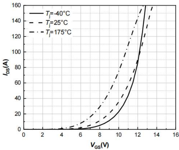
Fig.7 I_{DS}(A) vs V_{GS} V_{DS}=20V
