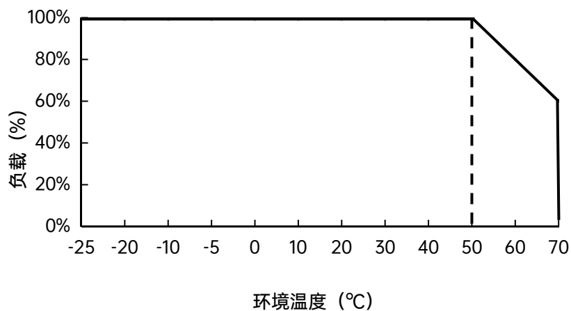
环境温度 VS 输出负载
