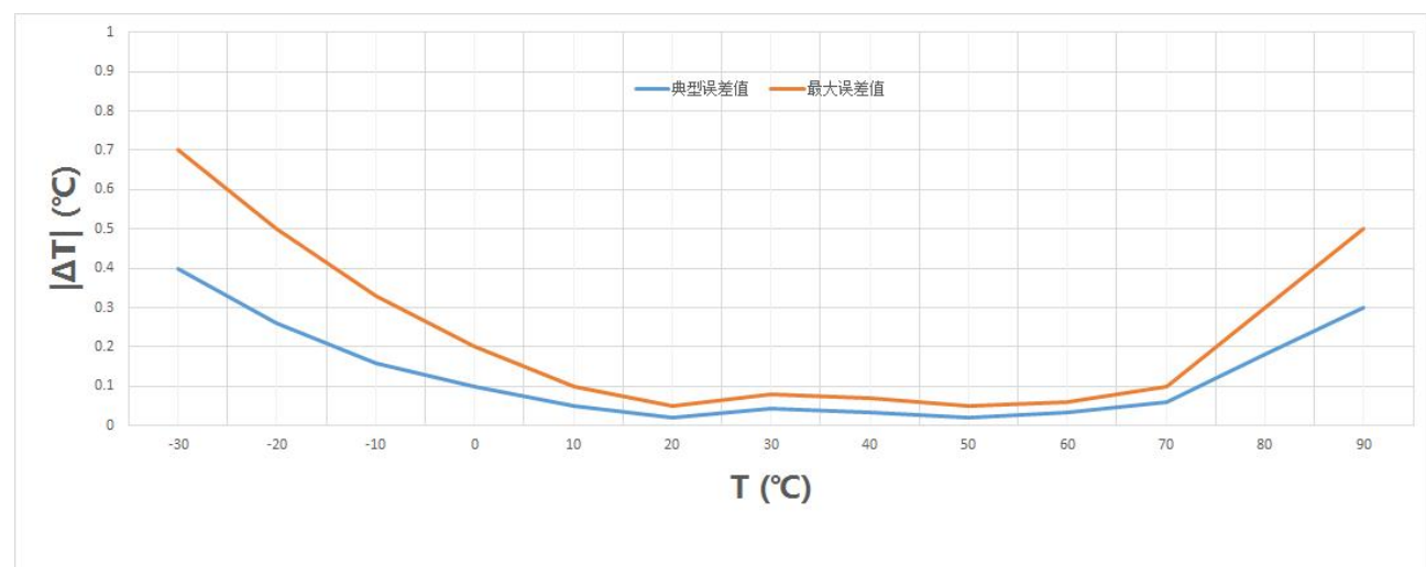
图 7-2 T1601Z 精度误差曲线
