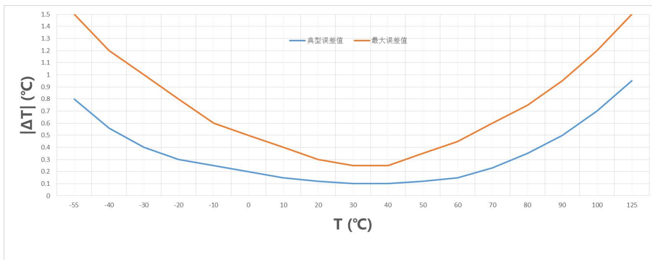
图 7-5 T1601B 精度误差曲线
