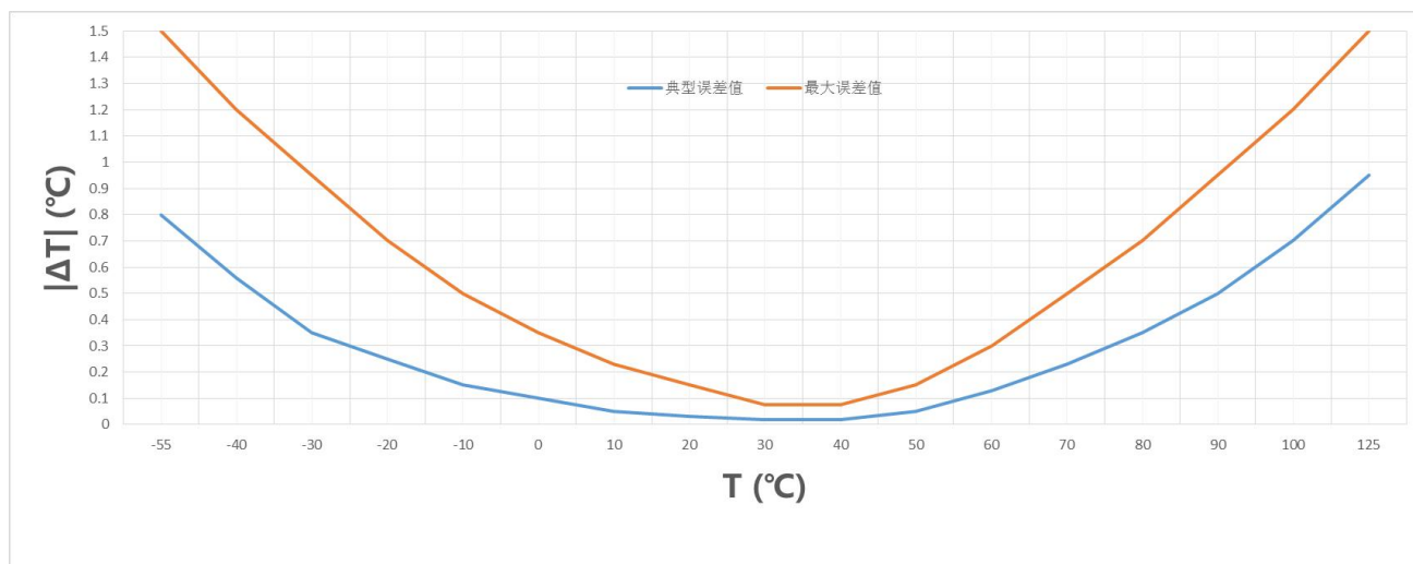
图 7-1 T1601 精度误差曲线
