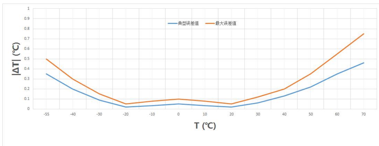
图 7-4 T1601P 精度误差曲线
