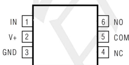
SOT363
