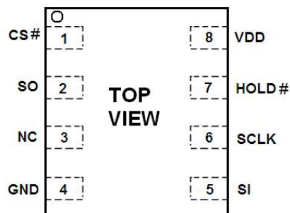
USON8 2X3
