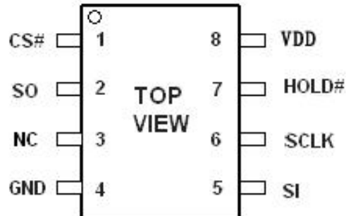
SOP8-A
