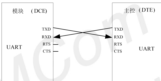
图 16: 串口连接图（NULL 模式）
