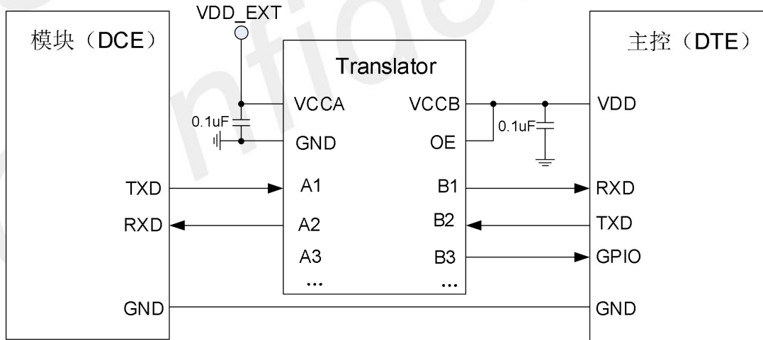
图 17: IC 电平转换参考电路
