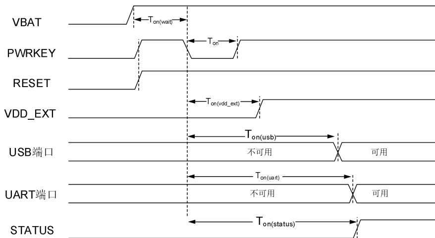
图 11: PWRKEY 开机时序
