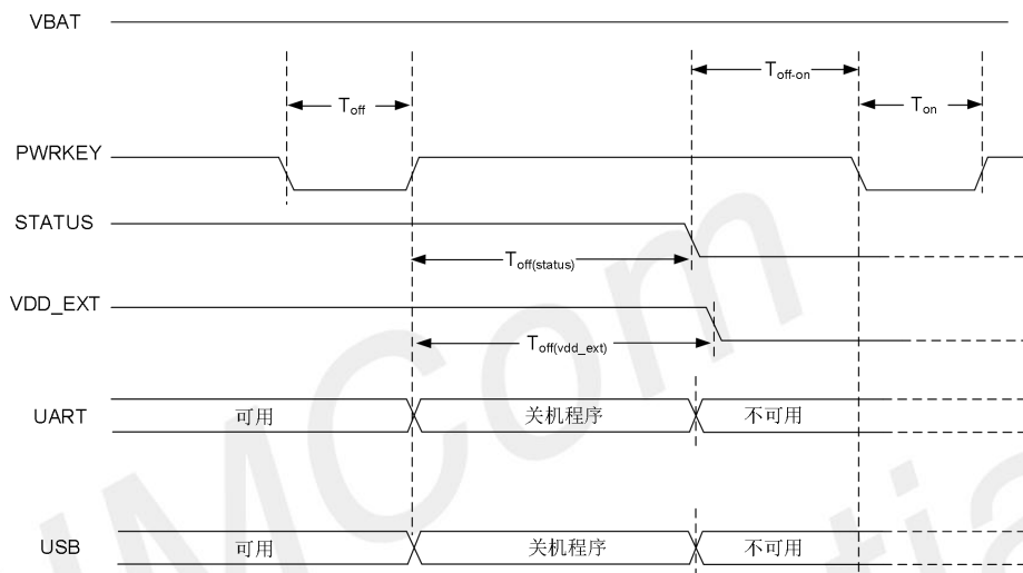
图 12: PWRKEY 关机时序
