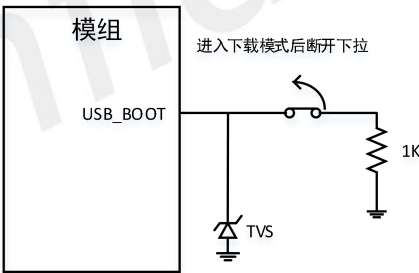
图 21: USB_BOOT 连接图
