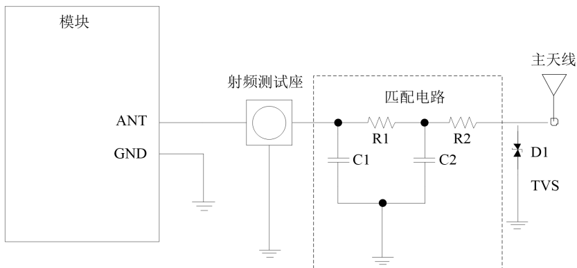
图 28：无源天线连接电路
