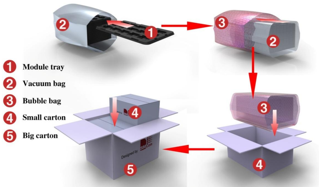
图 34：托盘包装示意图
