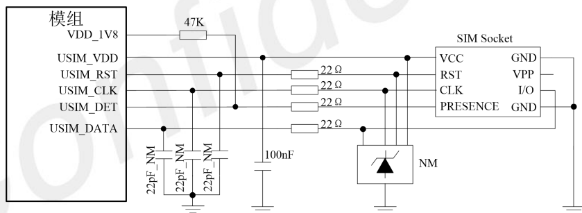
图 24: USIM 接口推荐电路(8PIN)
