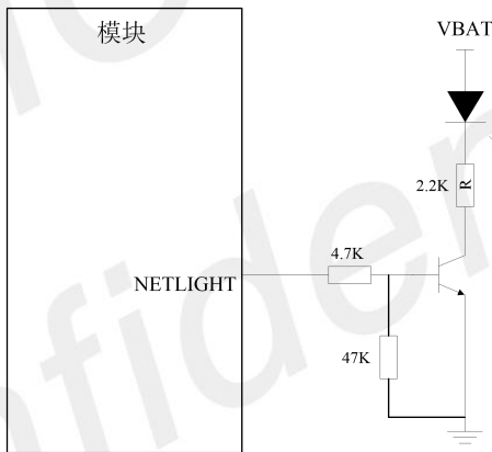
图 26: NETLIGHT 参考电路
