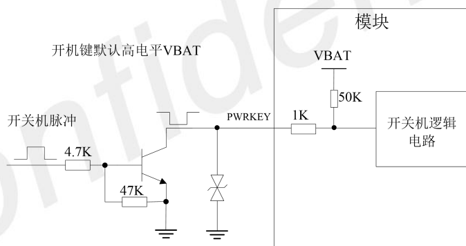
图 10: 开关机参考电路
