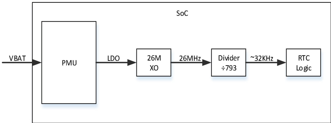
图 27: A7680C RTC 框图
