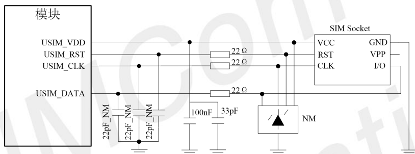
图 23: USIM 接口推荐电路
