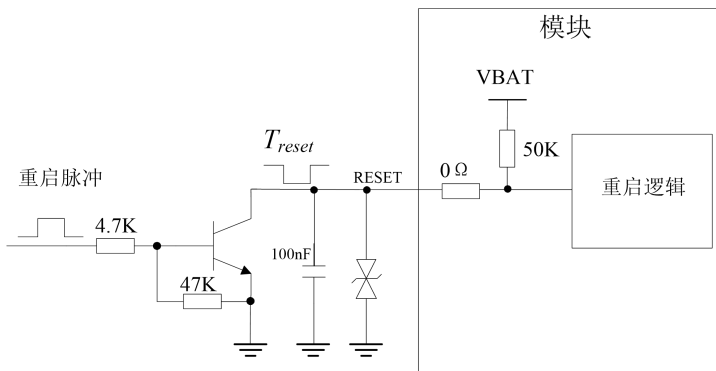
图 13: 复位推荐电路
