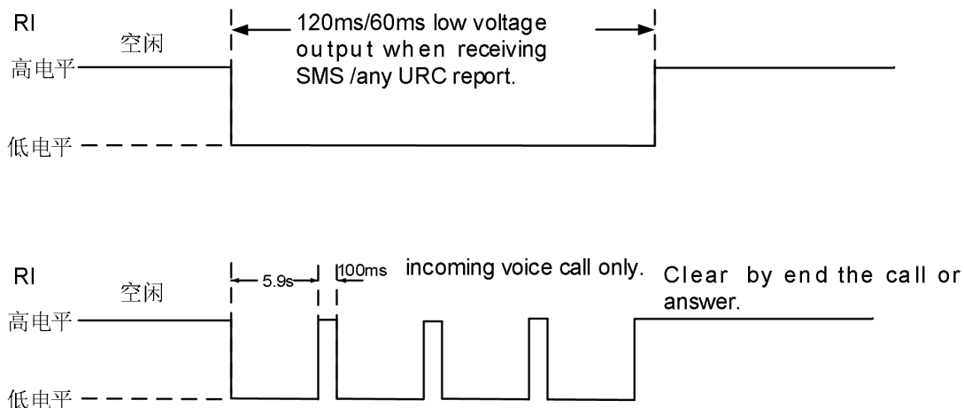
图 19: RI 上的电平变化(短信, URC, Incoming call)
