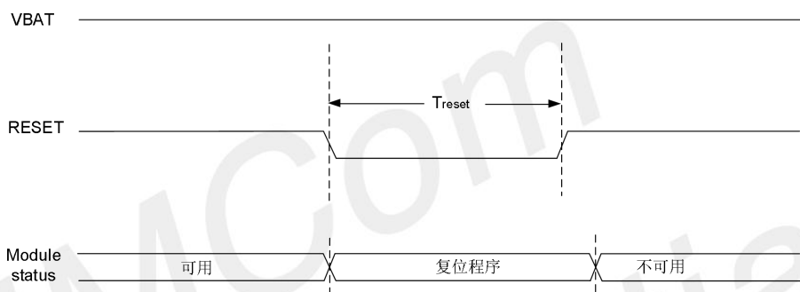
图 14: 复位时序
