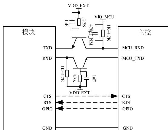
图 18: 三极管电平转换电路
