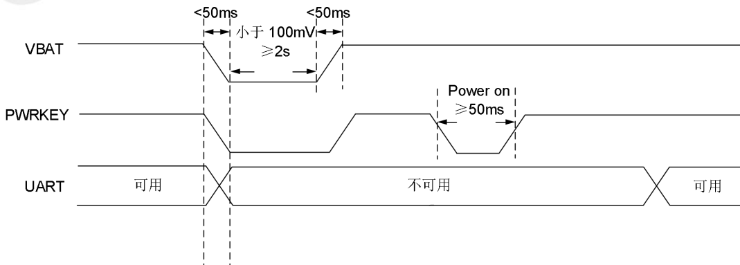
图 9：下电以及上电重启时序
