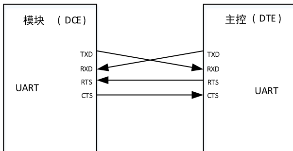
图 15: 串口连接图（全功能模式）
