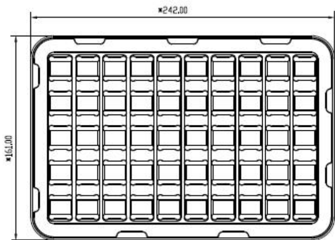
图 35：托盘尺寸图
