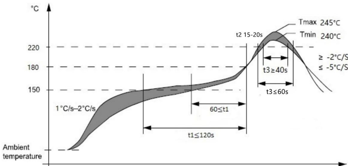
图 32: 推荐的焊炉温曲线图（无铅）
