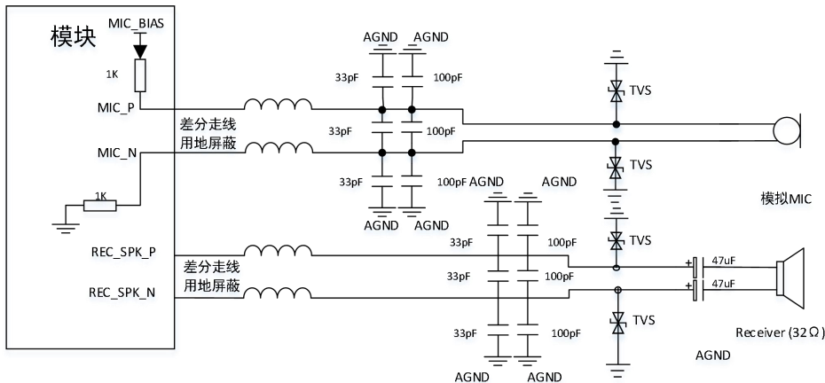
图 25: 模拟音频接口推荐电路
