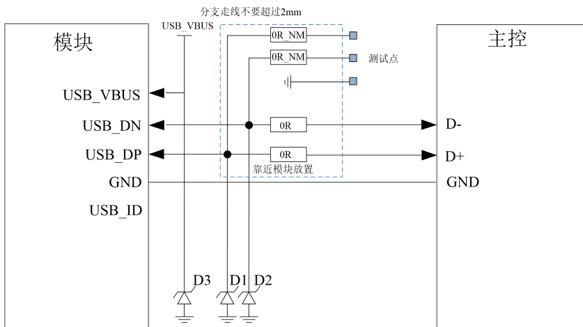
图 20: USB 连接图
