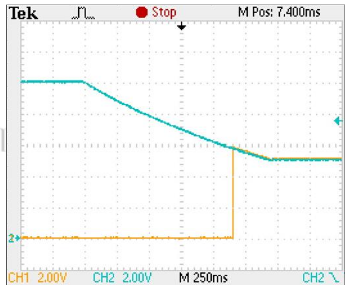
VIN falling waveform
