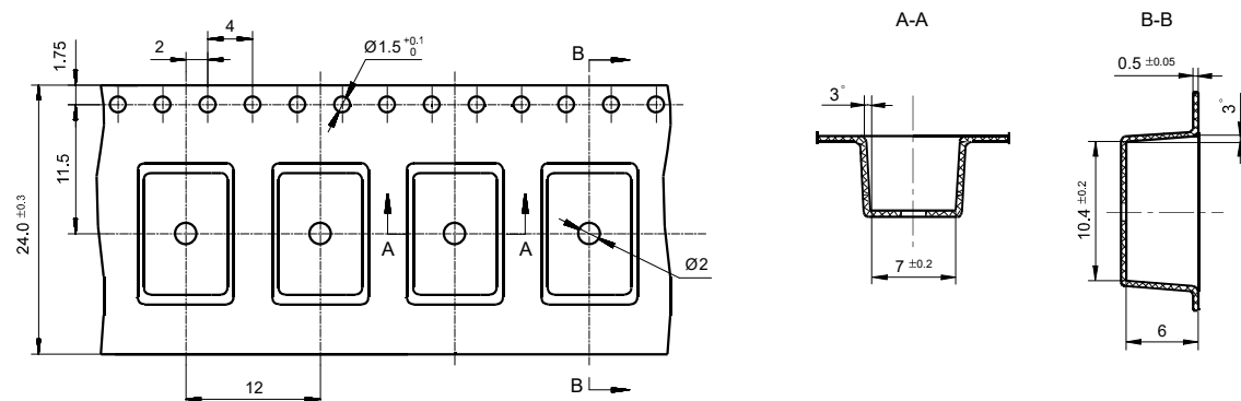
載帶外形圖 (S1型: 短腳表面貼裝型)
