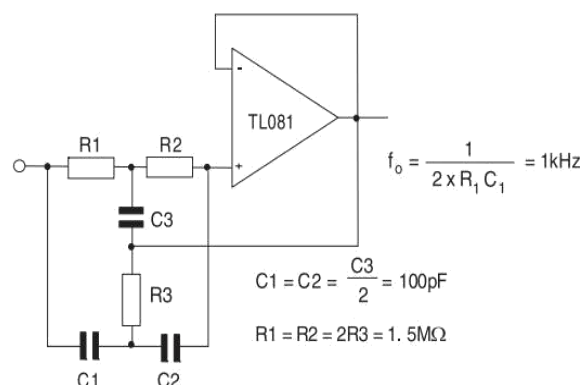
高 Q 阶式滤波器
