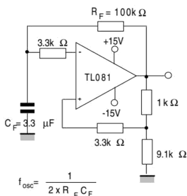
0.5Hz 方波振荡器
