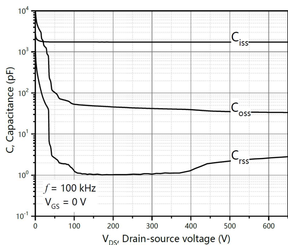
Typ. capacitances
