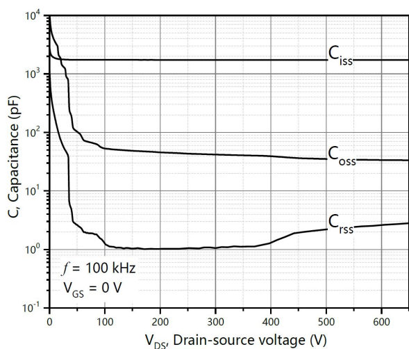
Typ. capacitances
