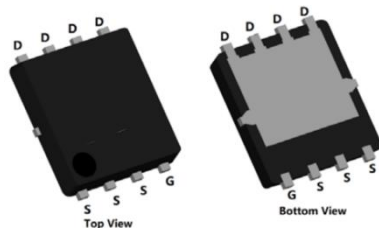
PDFN5X6-8L
