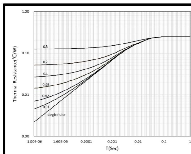
图 8 瞬态热阻抗
