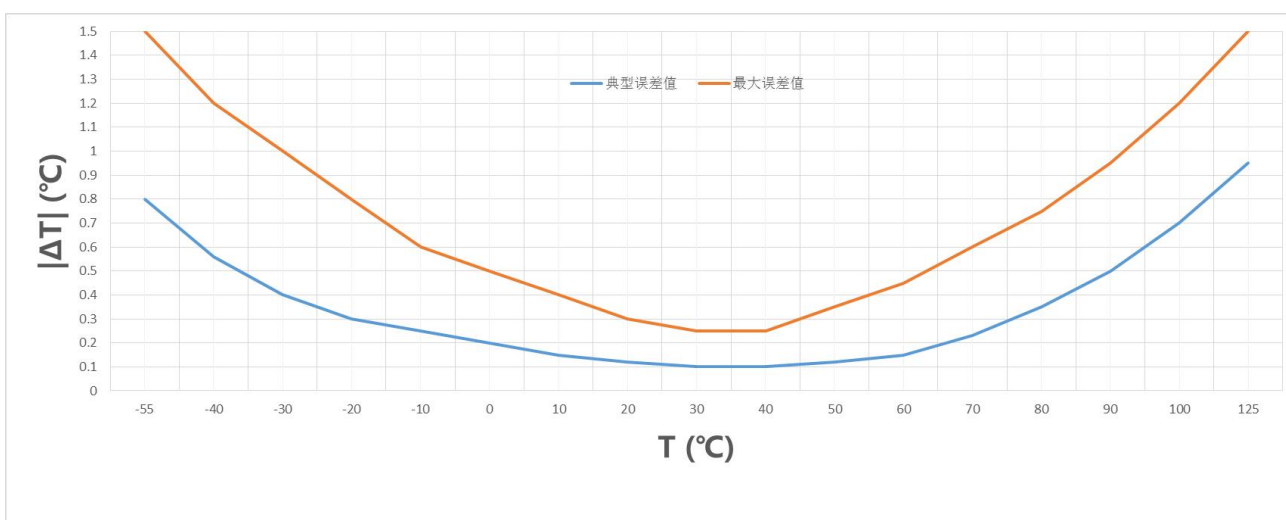
图 7-5 T117B-OW 精度误差曲线
