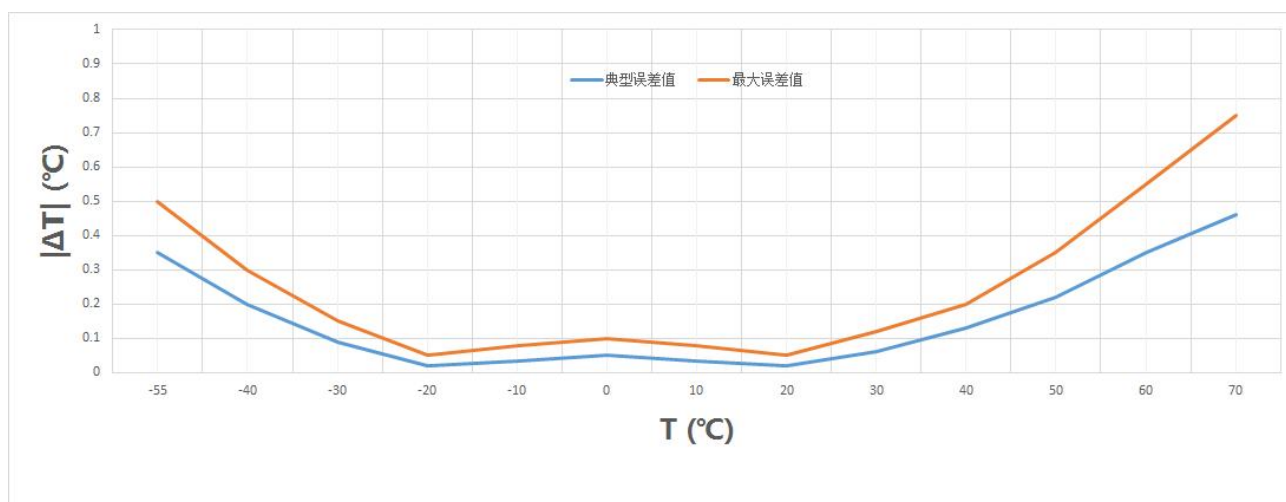
图 7-4 T117P-OW 精度误差曲线
