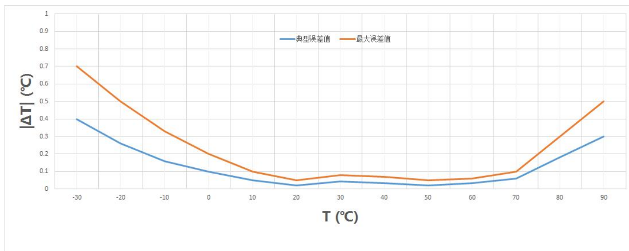
图 7-3 T117W-OW 精度误差曲线
