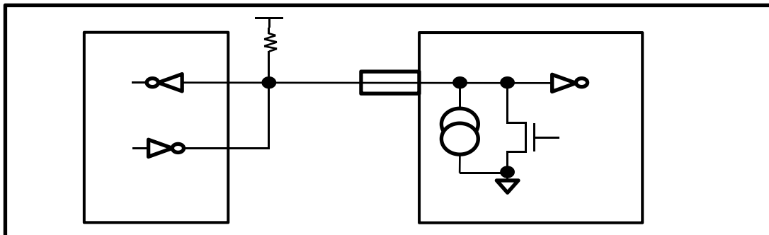
图 11.1 单总线硬件配置
