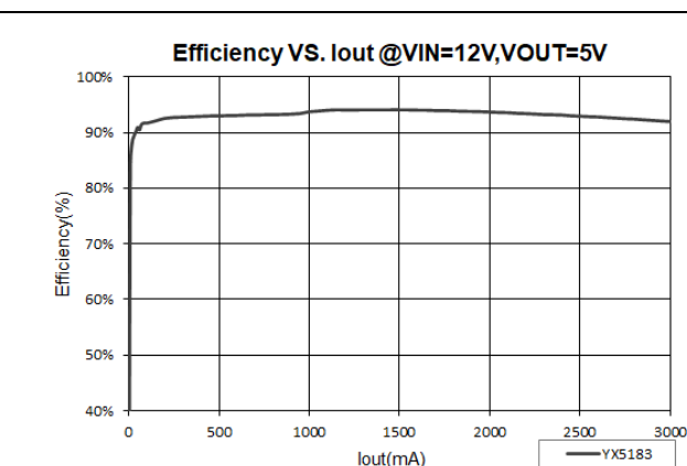
效率 VS 输出电流
