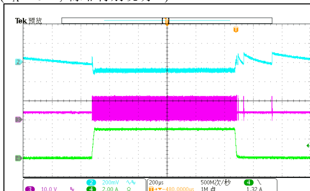
瞬态响应
