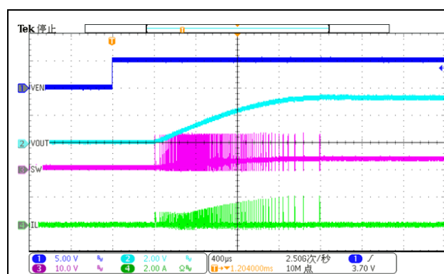
轻载EN启动
