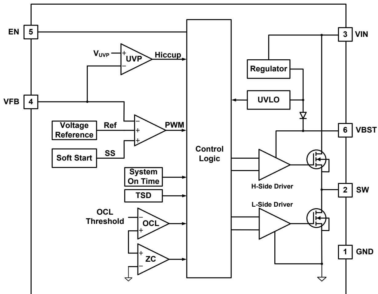
逻辑框图
