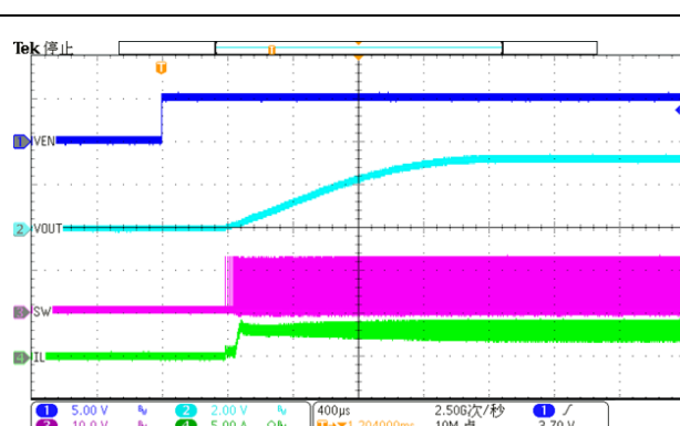
重载EN启动
