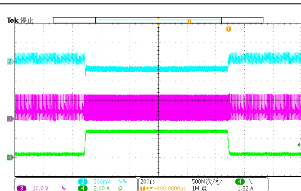
瞬态响应
