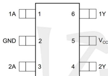
SOT363
