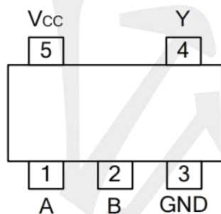
SOT23-5
