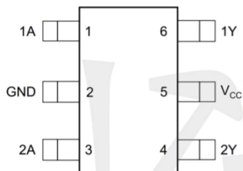
SOT363
