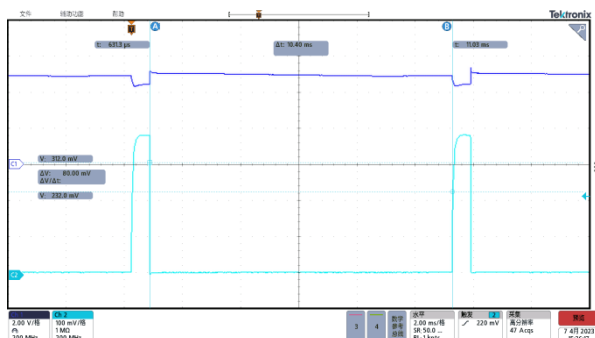
图 9: 过流保护恢复时间, T_{REC\_OCP}=10.40ms
