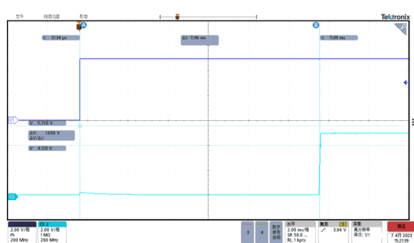
图 6: 上电去抖动时间, T_{DEB}=11.96ms
