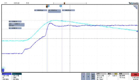
图 7: 过压保护响应时间, T_{OFF\_RES}=43.3ns
