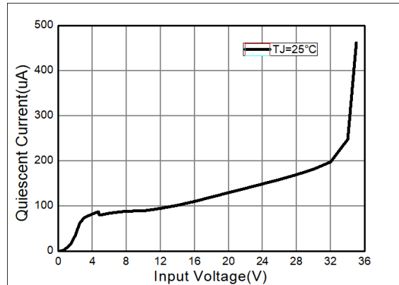
图 2: 静态电流 vs 输入电压
