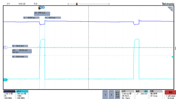
图 8: 过流保护去抖动时间, T_{OCP}=640us
