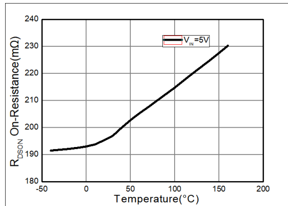
图 4: 导通电阻 vs 温度
