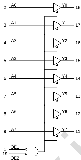
图 1 逻辑符号
