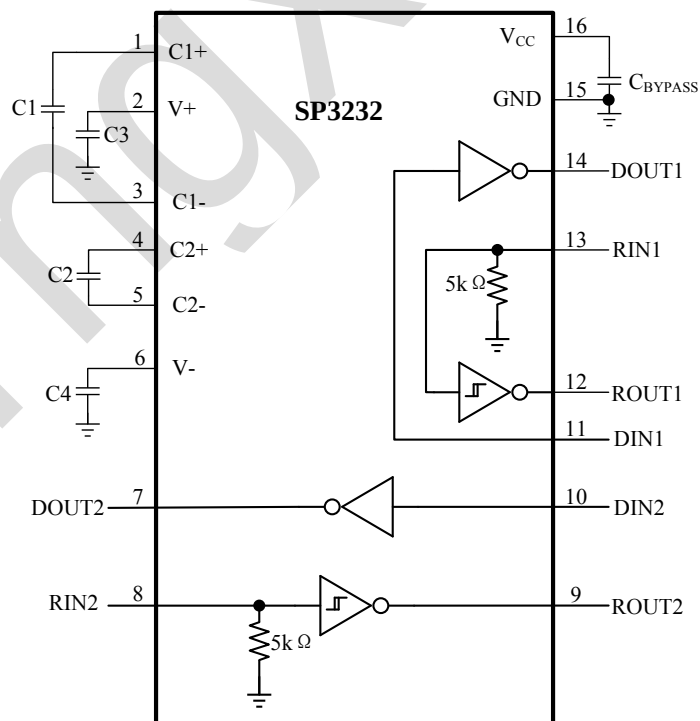
SP3232 典型应用图
