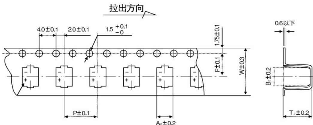
Fig.1 (Φ4 ~ Ø10)
