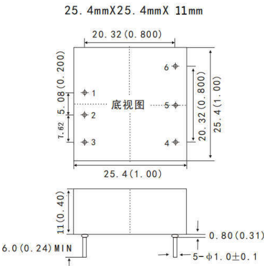
T_YMD-10WR3E 管脚定义
