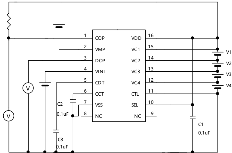
测定电路 3
