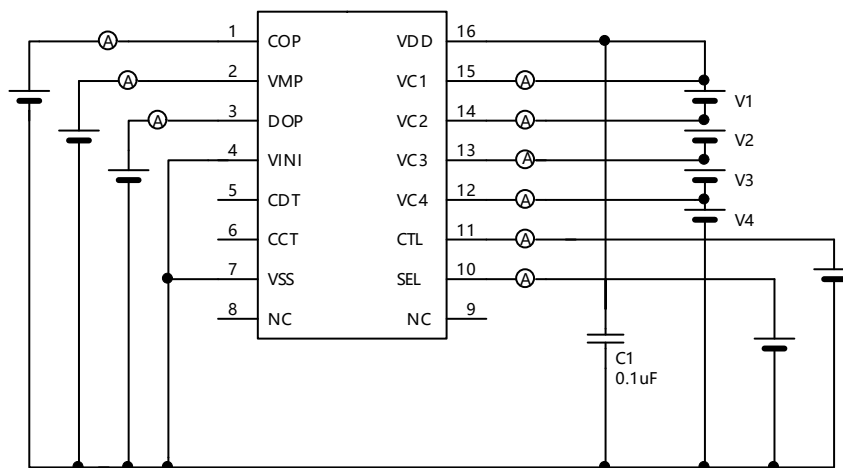
测定电路 5
