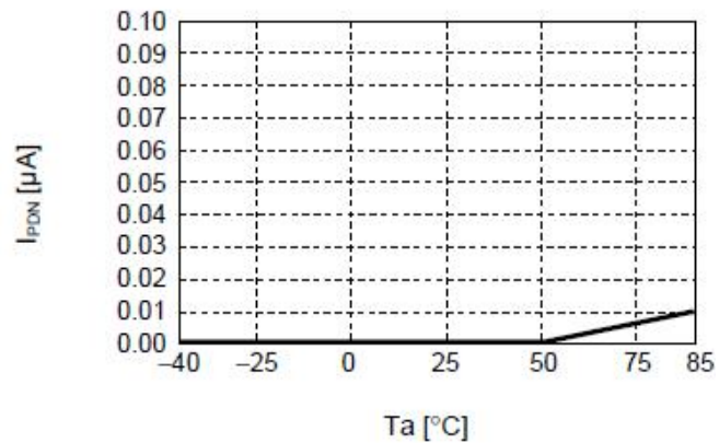
4. I_{PDN}-T_a
