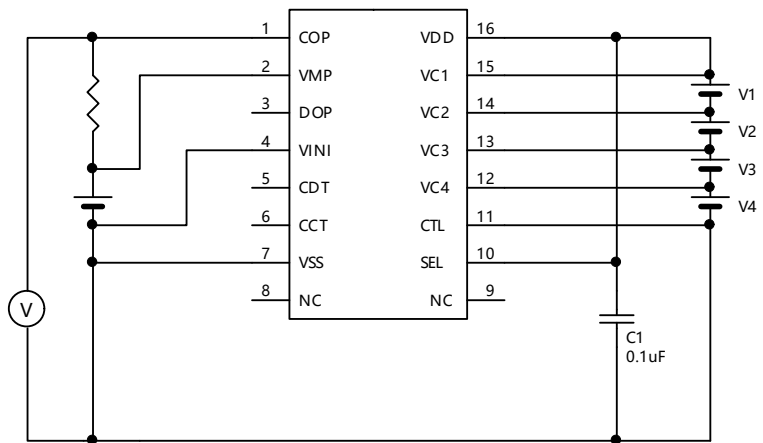
测定电路 4
