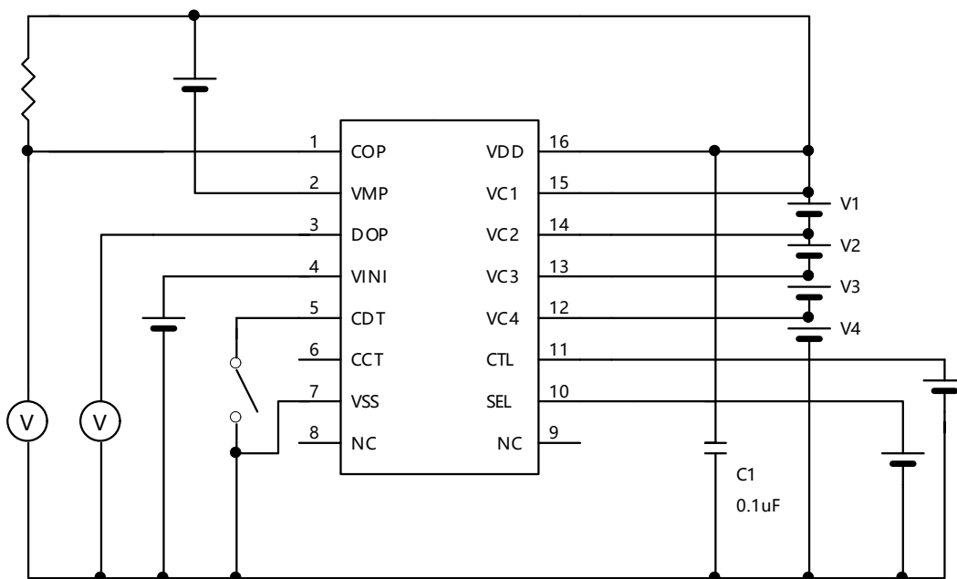
测定电路 2
