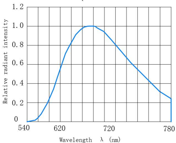
光谱分布曲线 Relative Spectral Distribution
