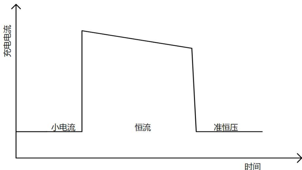
图 4 充电过程
