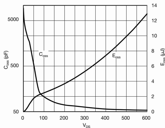
Fig. 6 - C_{oss} and E_{oss} vs. V_{DS}
