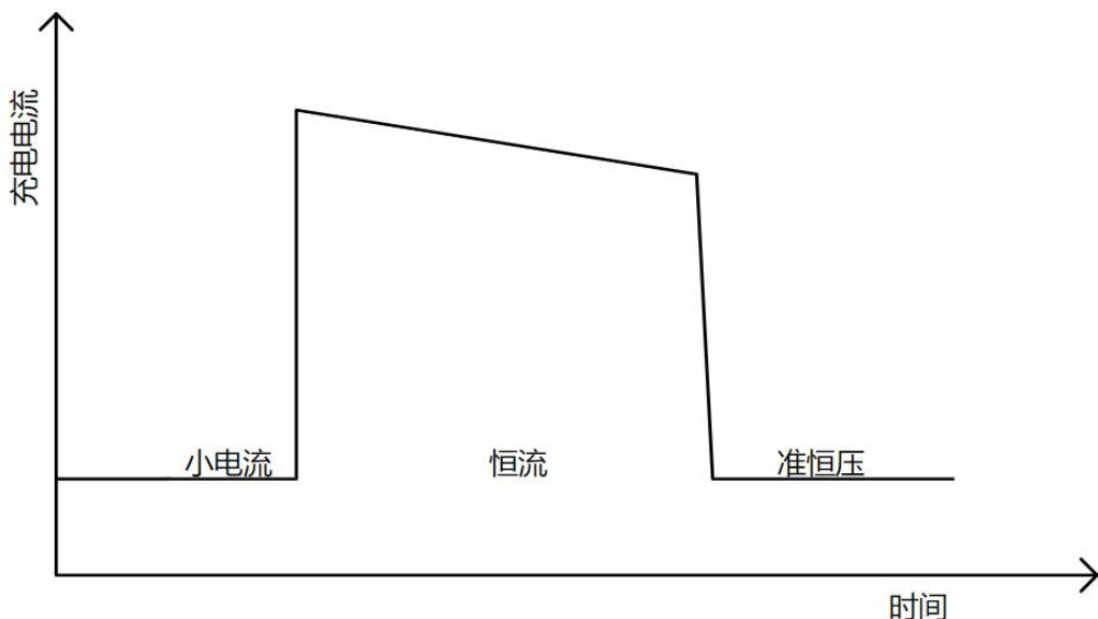
图 4 充电过程
