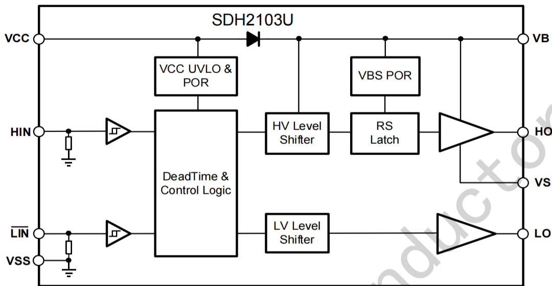
图 7-1 SDH2103U的功能框图
