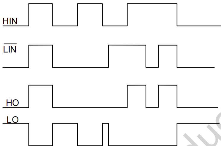
图6-1 SDH2103U 输入输出时序波形
