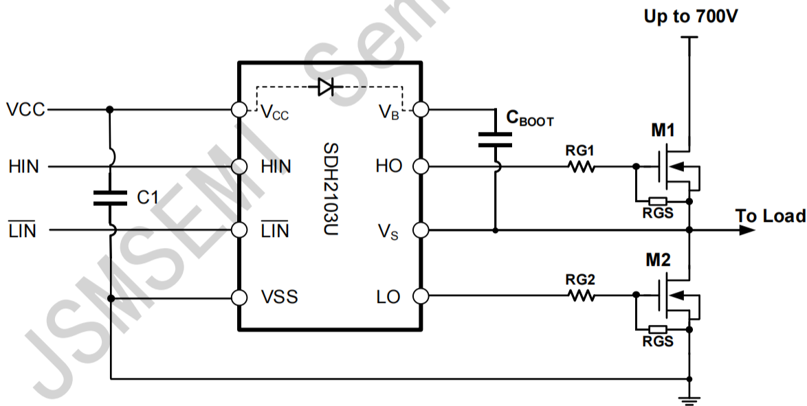
图 7-2 SDH2103U典型应用电路图
