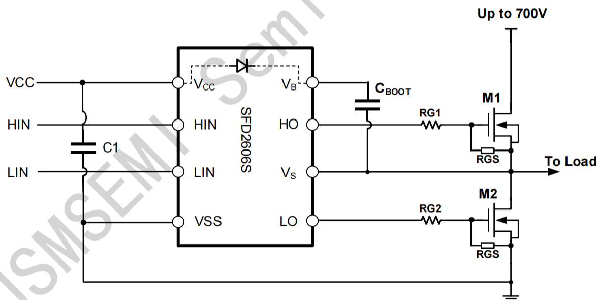
图 7-2 SFD2606S典型应用电路图
