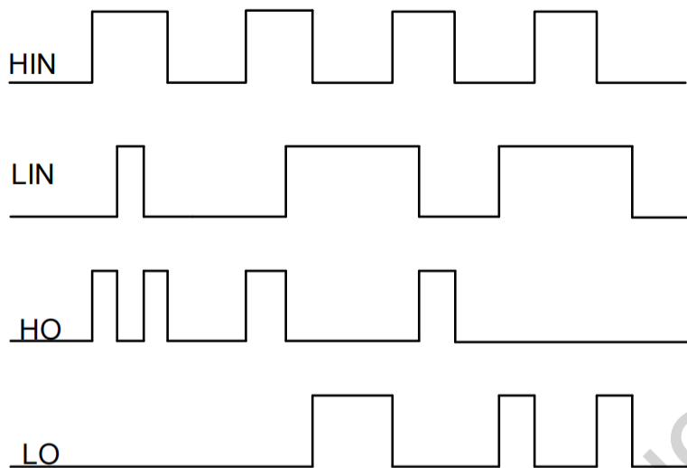
图 6-1 SFD2606S输入输出时序波形
