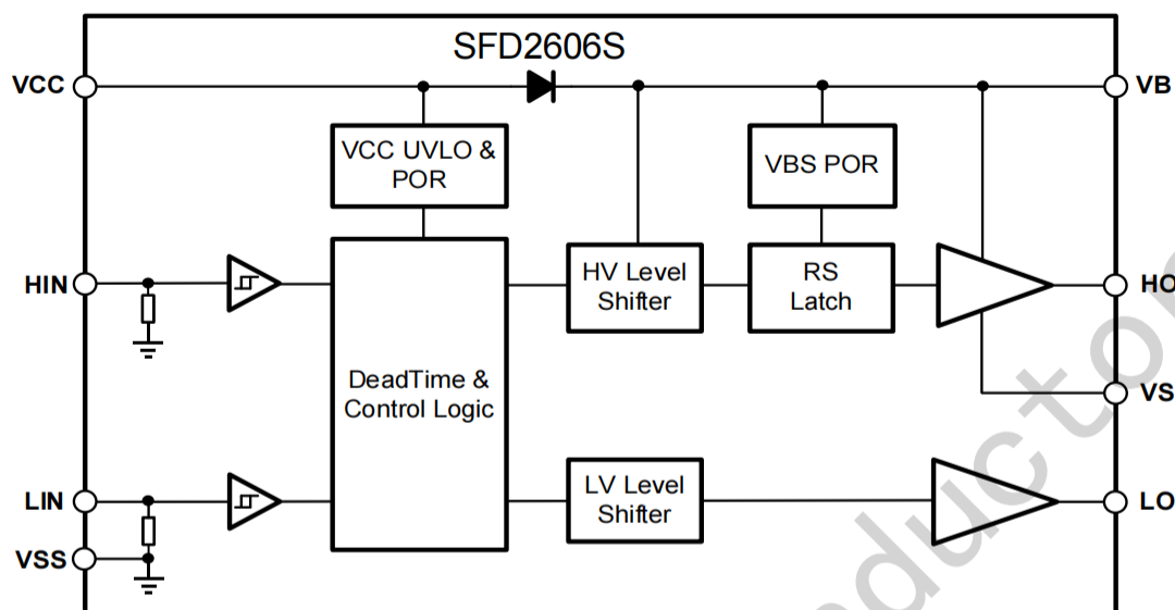
图 7-1 SFD2606S的功能框图
