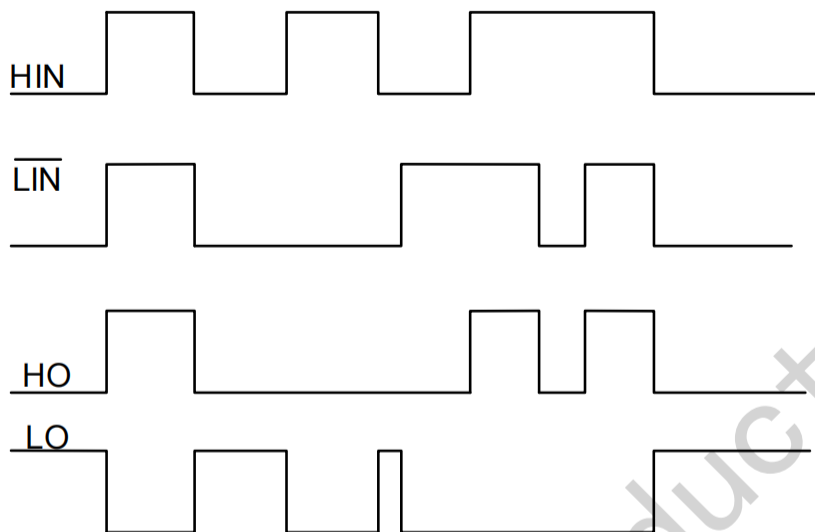
图 6-1 U3115S输入输出时序波形
