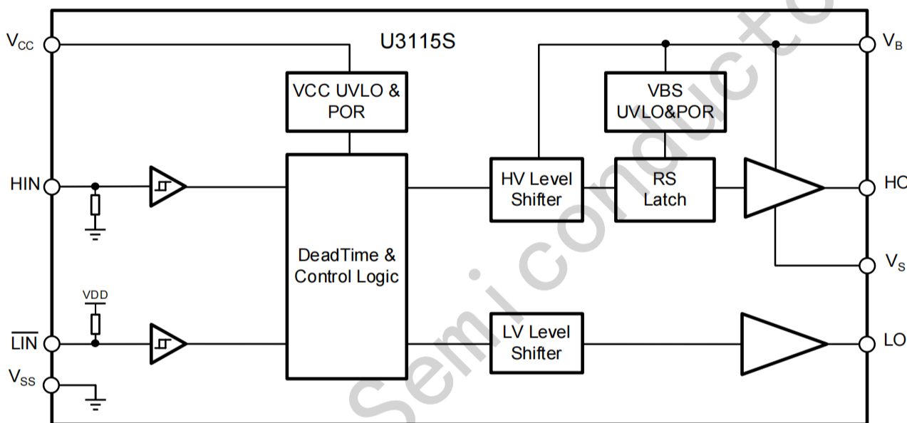
图 7-1 U3115S功能框图
