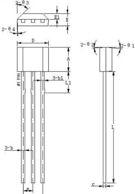
TO-92S-A1/A2 TO-92S-A1
