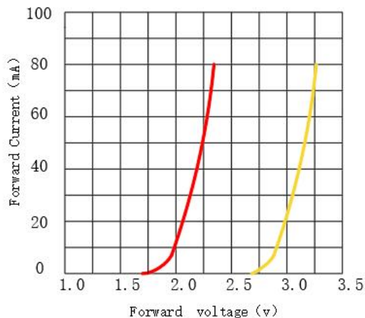
伏安特性 Volt ampere characteristic
