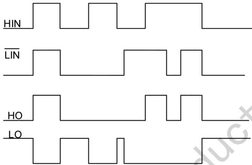
图 6-1 JSM2203S输入输出时序波形
