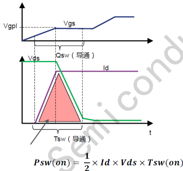
图 8-3 阻性负载条件下的 MOS 开关损耗
