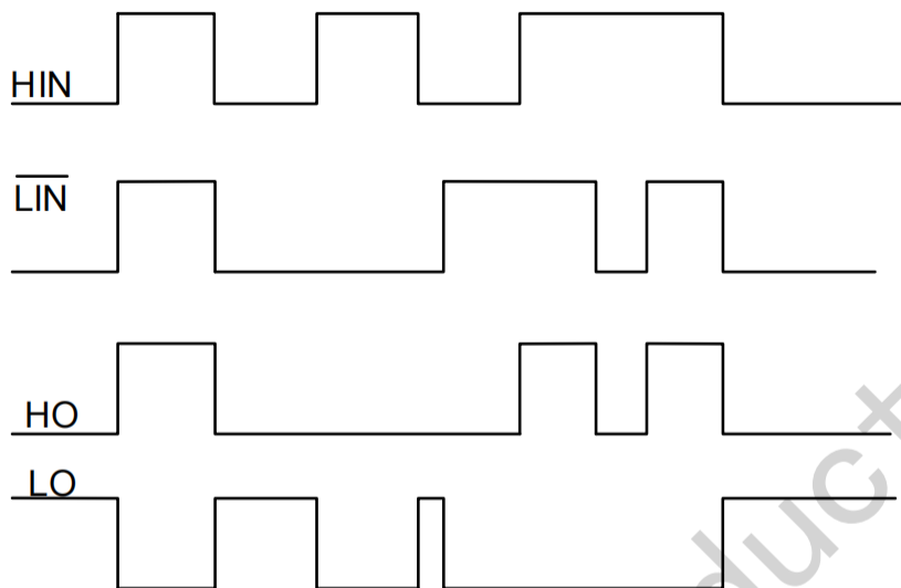
图 6-1 JSM2103S输入输出时序波形
