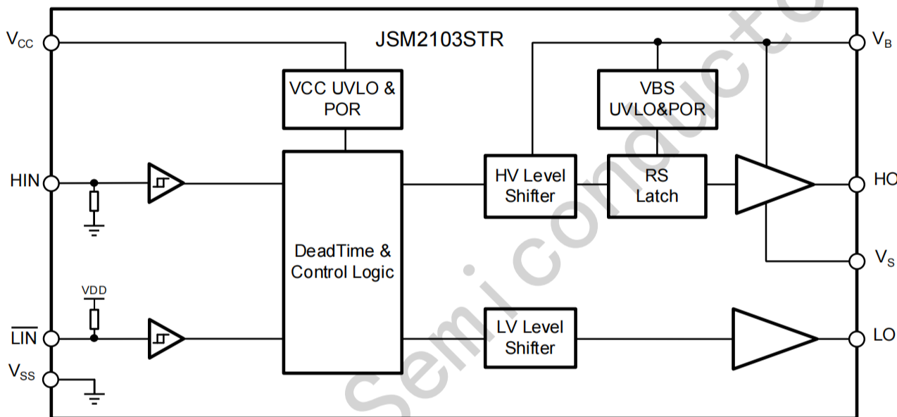
图 7-1 JSM2103S功能框图
