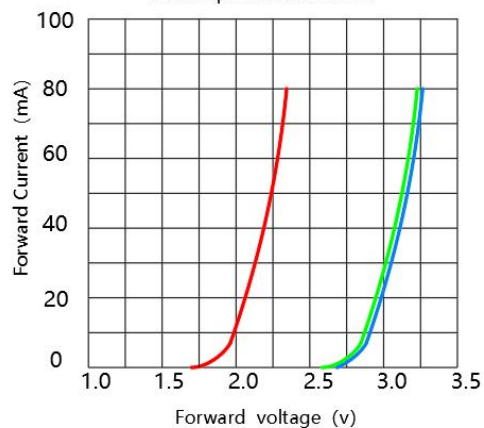
伏安特性 Volt ampere characteristic
