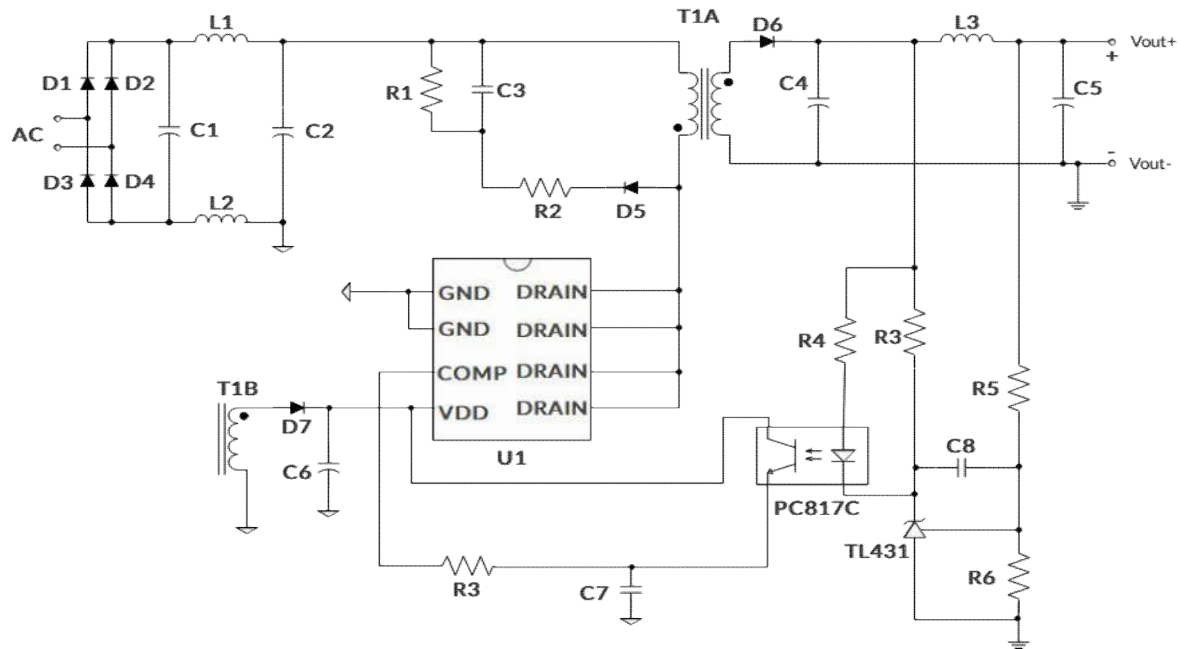
图 2 典型应用图
