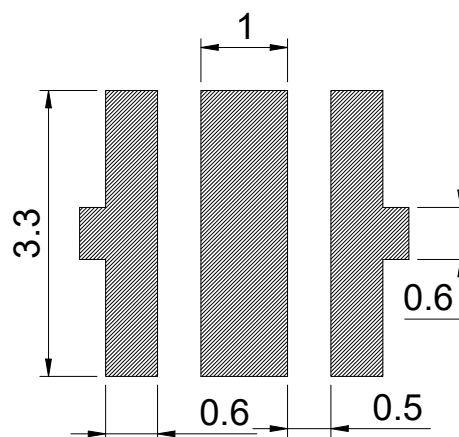
焊盘建议图
