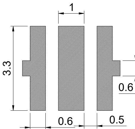
焊盘建议图
