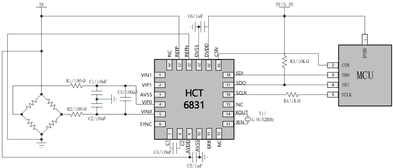
Figure 8-1 HCT6831 应用图 1
