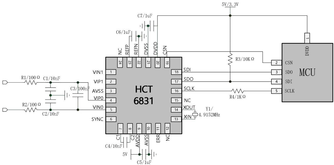
Figure 8-2 HCT6831 应用图 2
