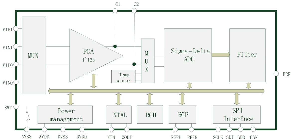
Figure 3-1 HCT6831 模块功能图
