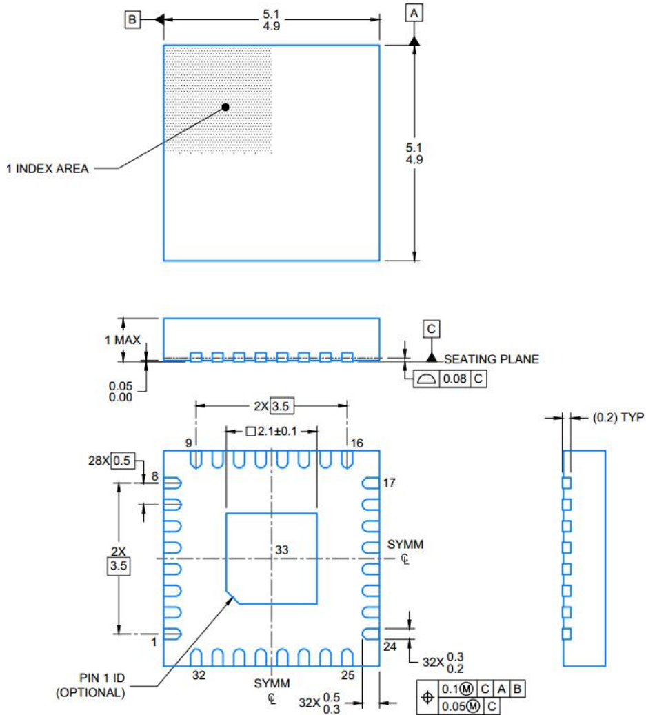
Figure 2-3 HCT6761Q/6763Q 封装尺寸
