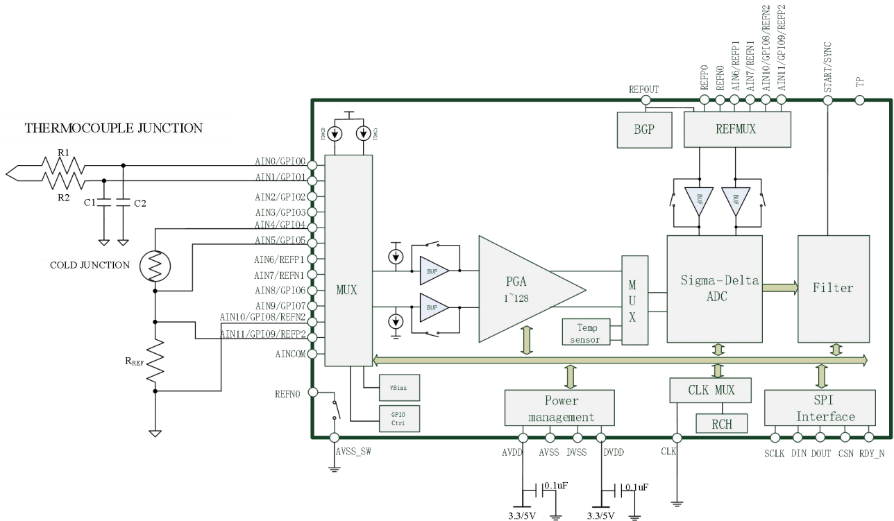
Figure 8-1 热电偶应用
