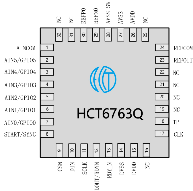
Figure 2-2 HCT6763Q 引脚分布图
