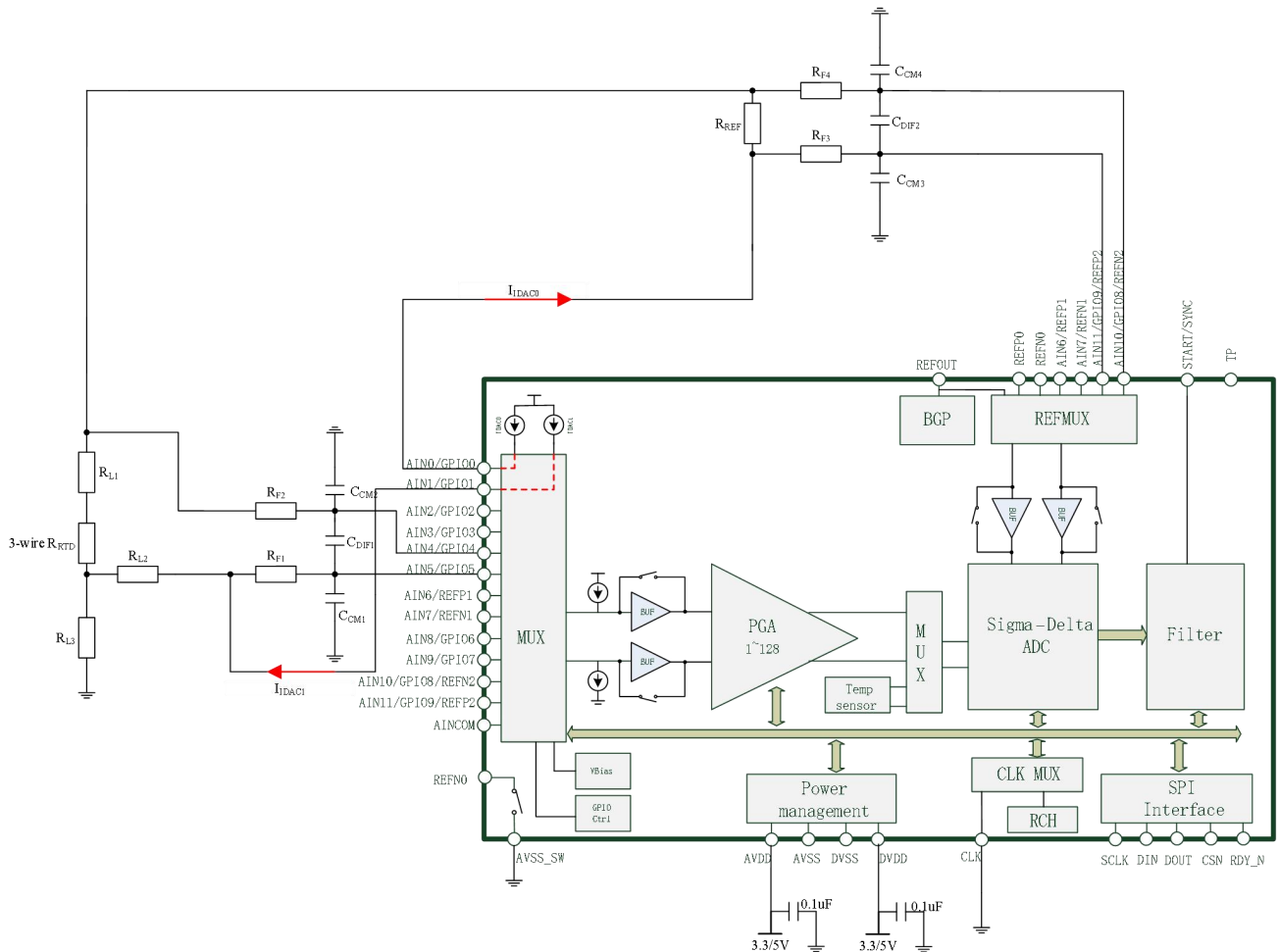
Figure 8-2 3 线 RTD 应用
