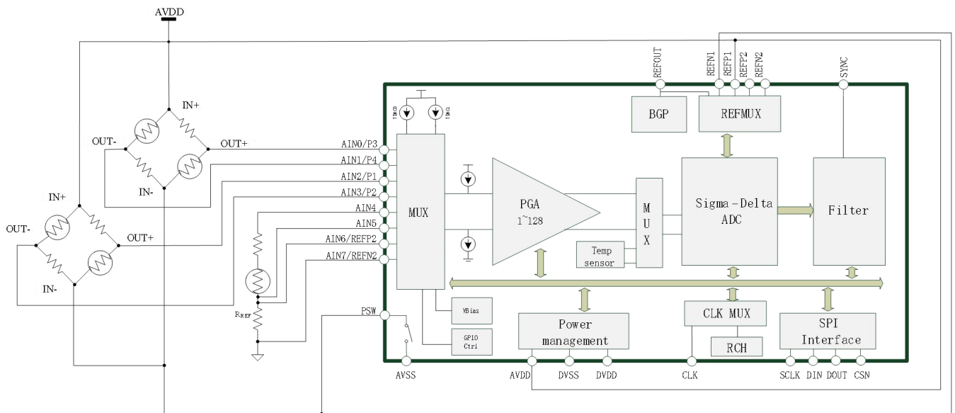
Figure 8-6 流量计应用
