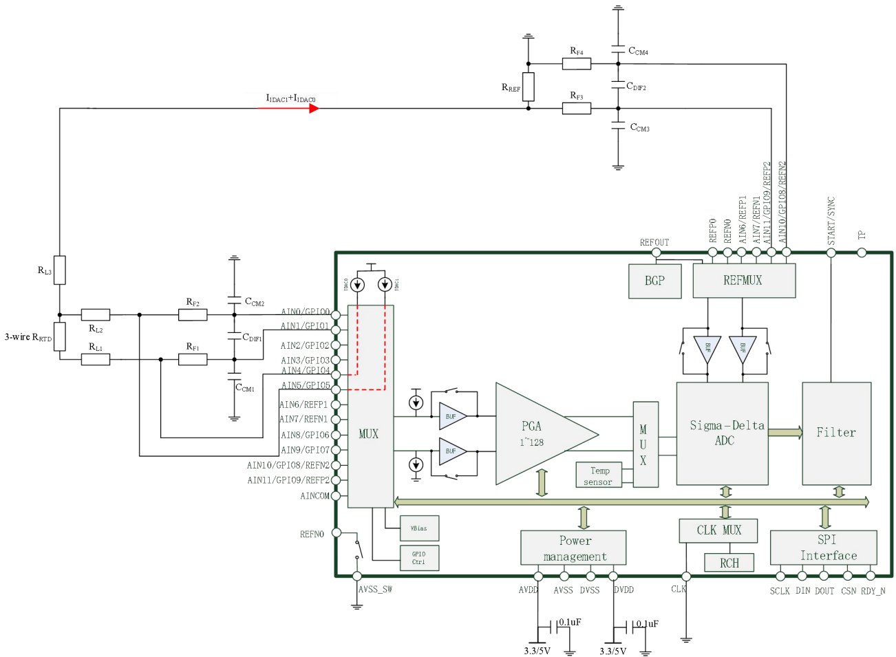
Figure 8-3 3 线 RTD 应用
