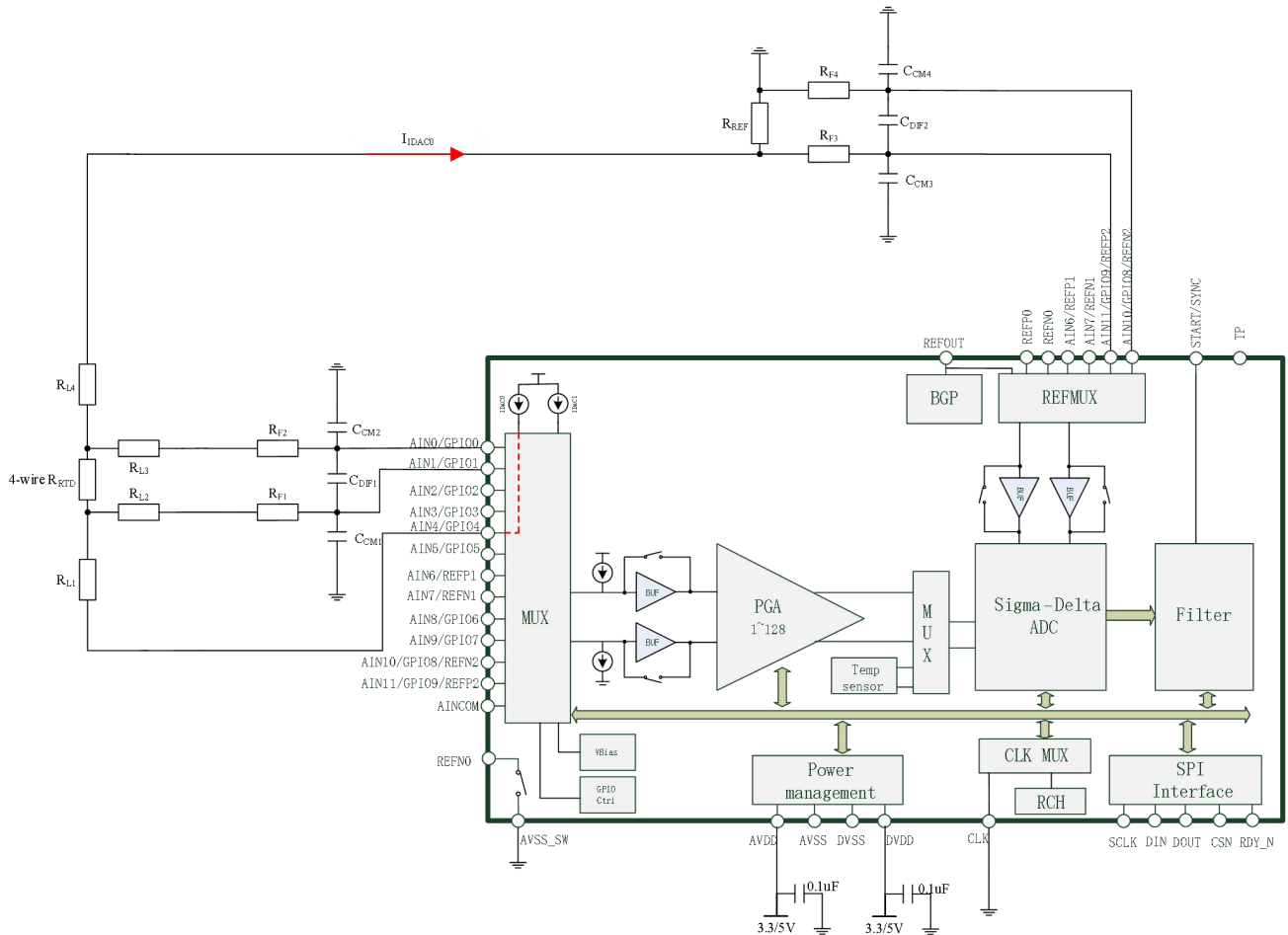
Figure 8-4 4 线 RTD 应用
