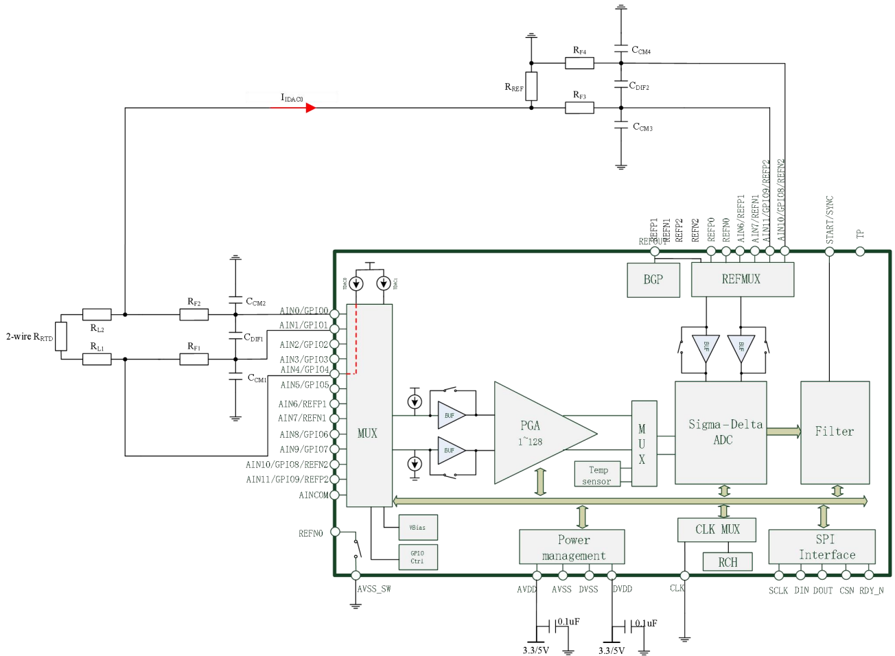
Figure 8-5 2 线 RTD 应用
