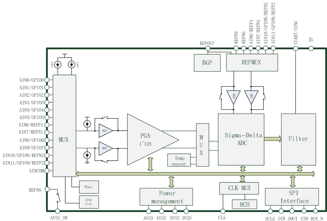
Figure 3-1 HCT676x 模块功能图
