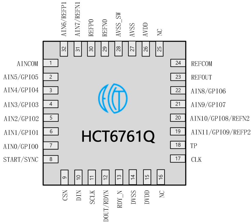
Figure 2-1 HCT6761/6761Q 引脚分布图
