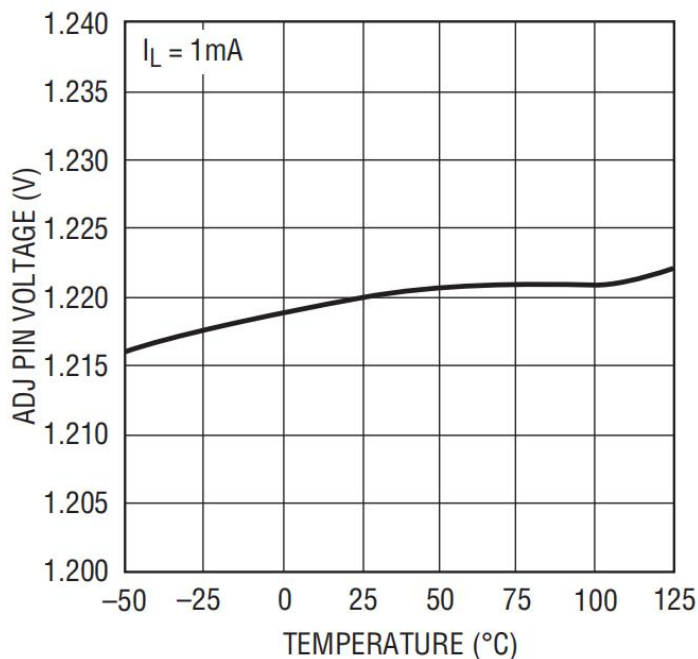
图 7 输出电压和温度关系曲线图 (LKP2872ST-ADJ)
