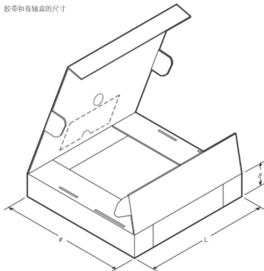
胶带和卷轴盒的尺寸
