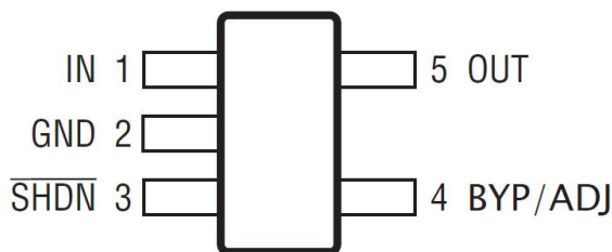
图 3 LKP2872ST 引脚排列图（顶视图）
