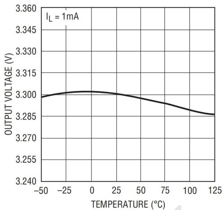
图5 输出电压和温度关系曲线图 ((LKP2872ST-33))
