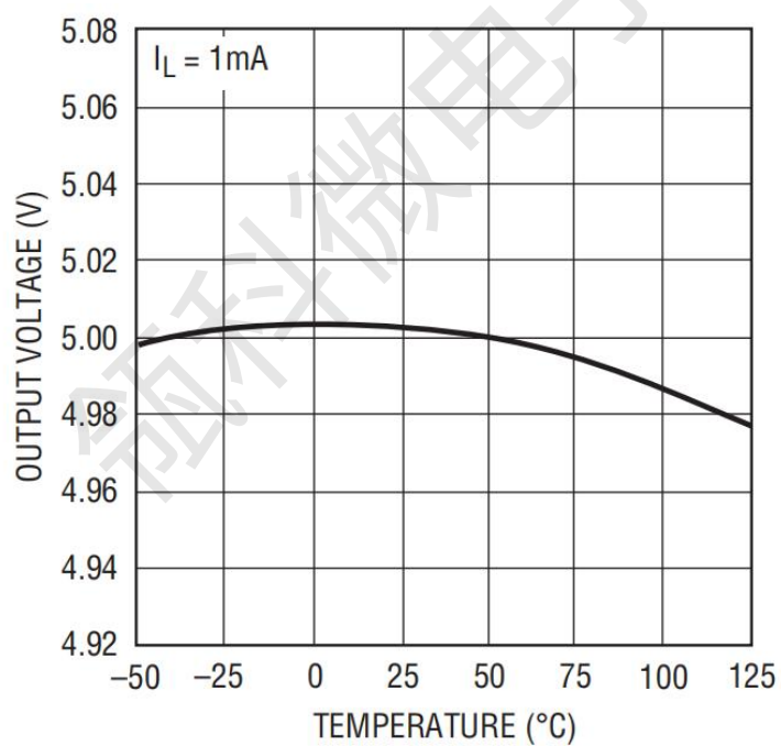
图6 输出电压和温度关系曲线图 ((LKP2872ST-5))
