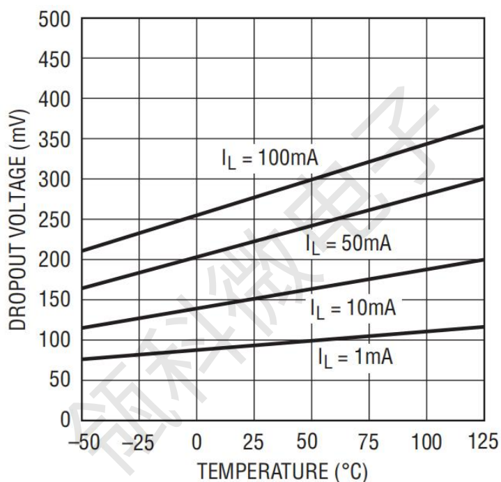
图 4 压差和负载电流&温度关系曲线图
