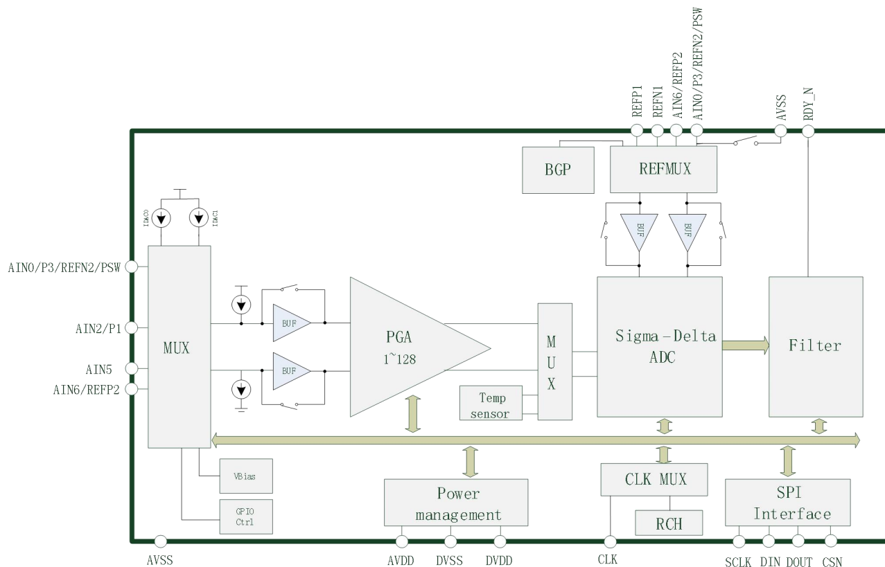
Figure 3-1 HCT6911 模块功能图
