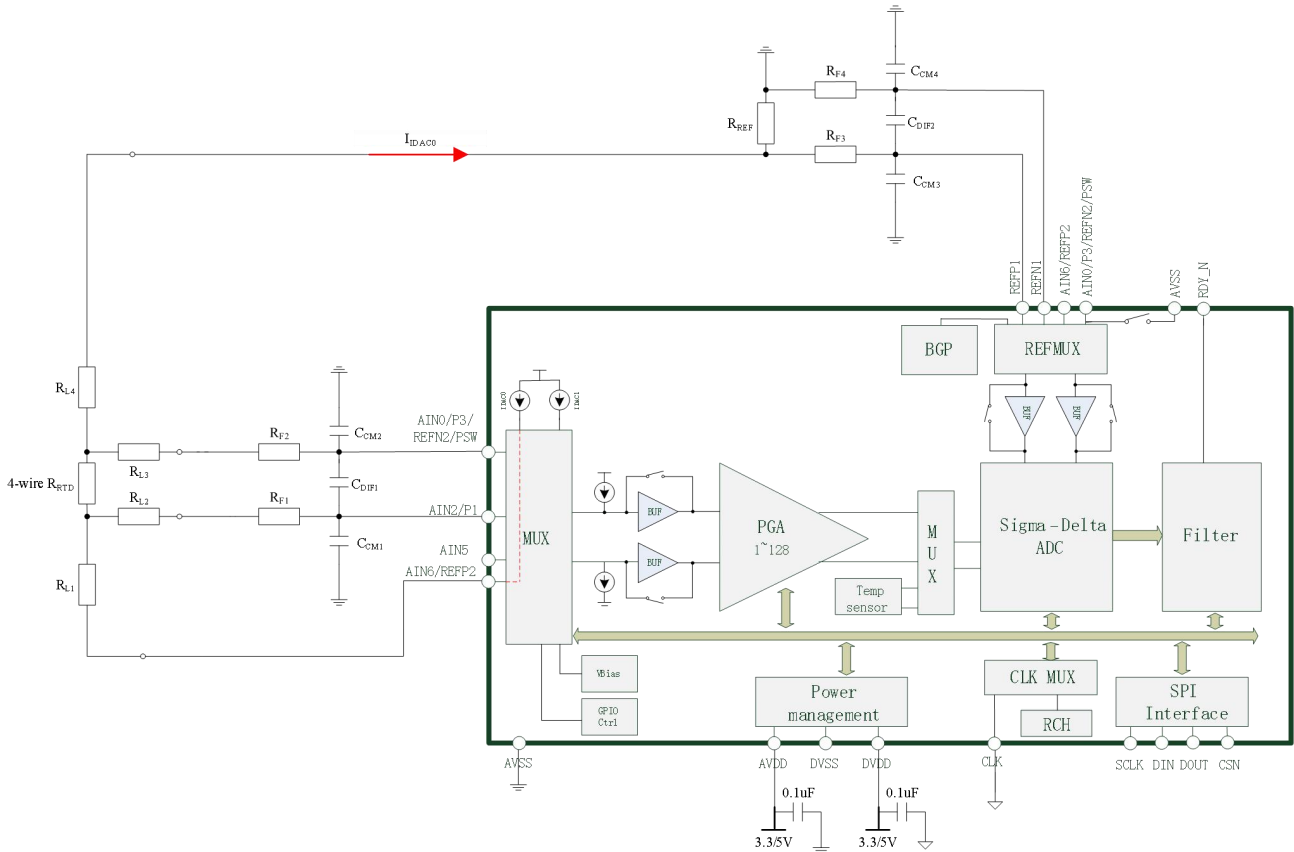
Figure 8-4 4 线 RTD 应用
