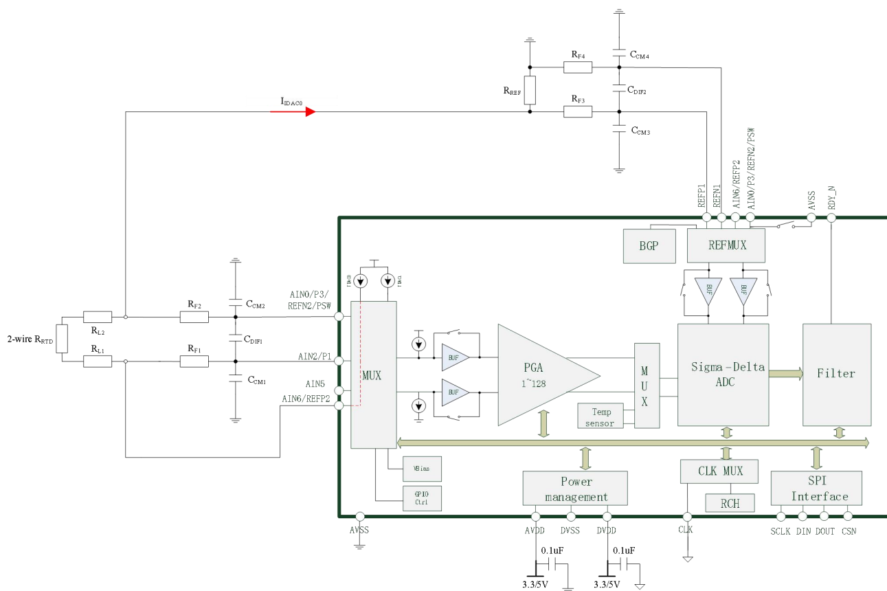
Figure 8-5 2 线 RTD 应用
