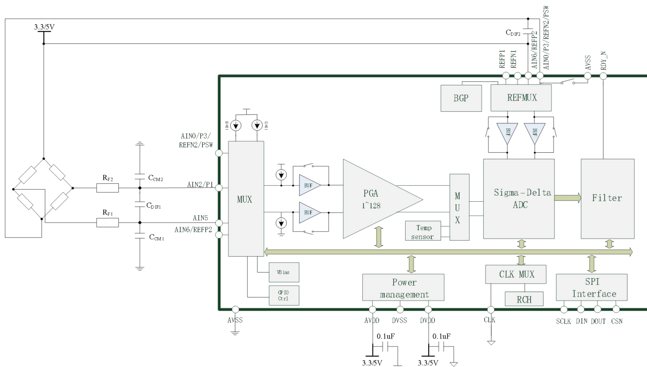
Figure 8-6 桥式传感器应用
