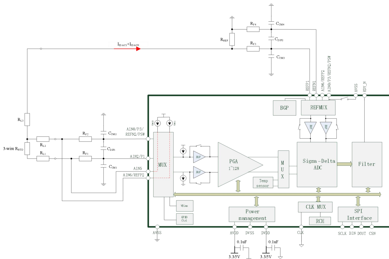
Figure 8-3 3 线 RTD 应用
