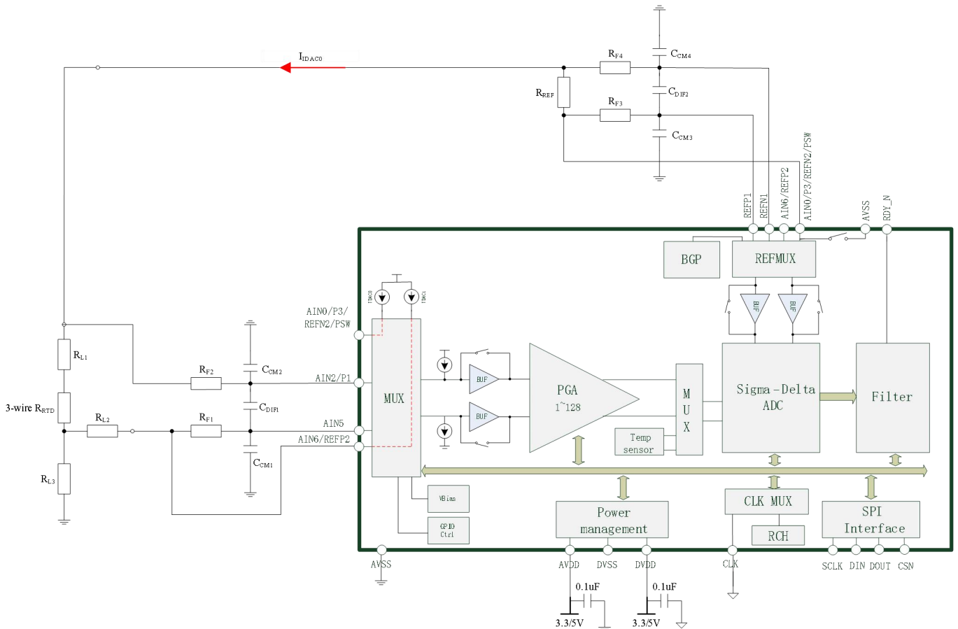
Figure 8-2 3 线 RTD 应用
