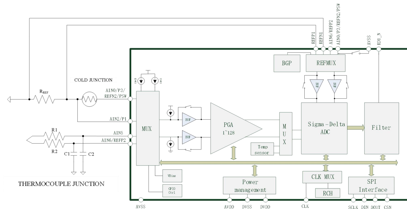
Figure 8-1 热电偶应用
