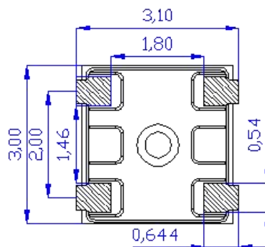
背面图
