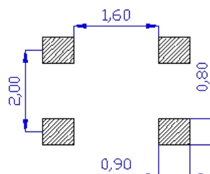
建议焊盘 仅供参考
