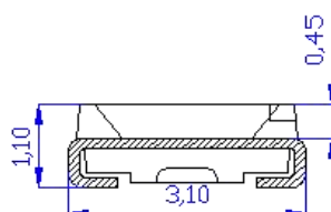
侧面图
