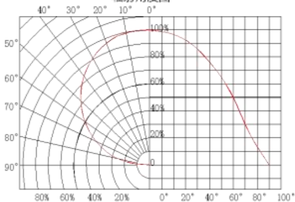
辐射角度图
