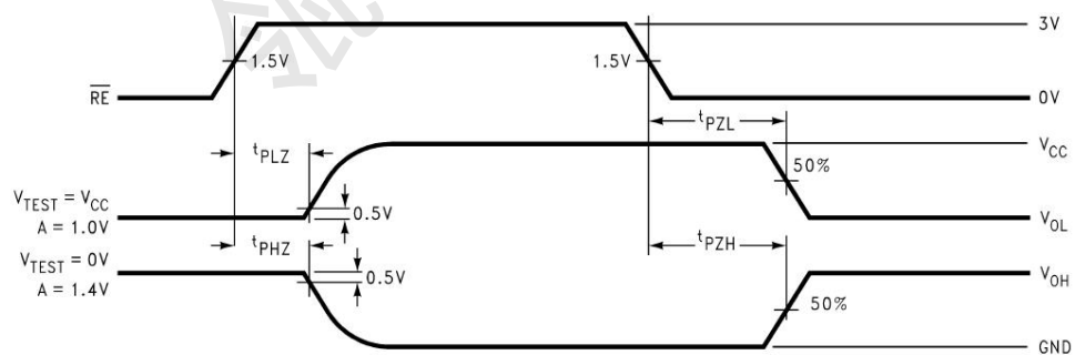
图 18 接收器三态延时波形图
