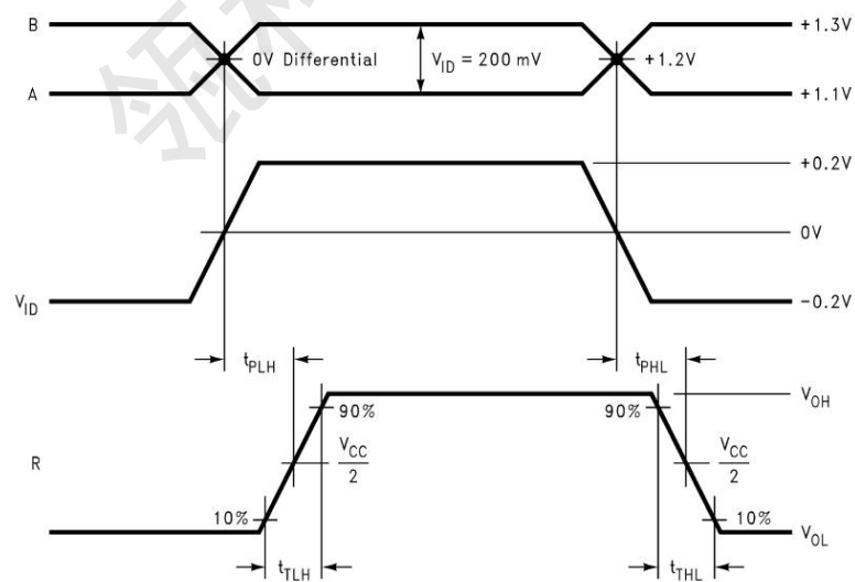
图 15 接收器模式 1 传输延时和传输时间波形图
