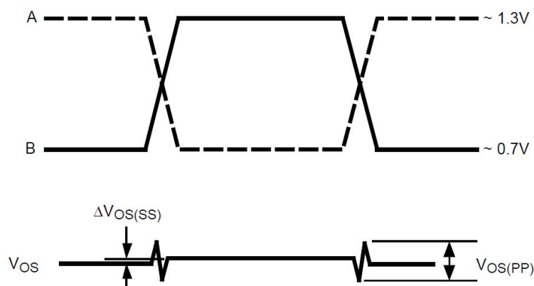
图 6 差分驱动波形图
