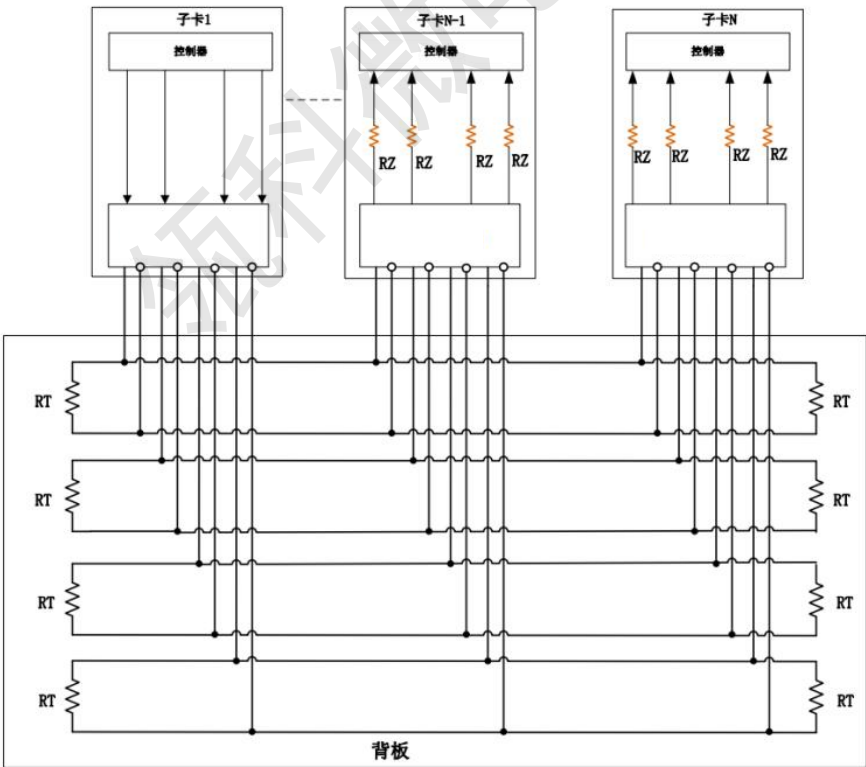
图 1 典型应用框图
