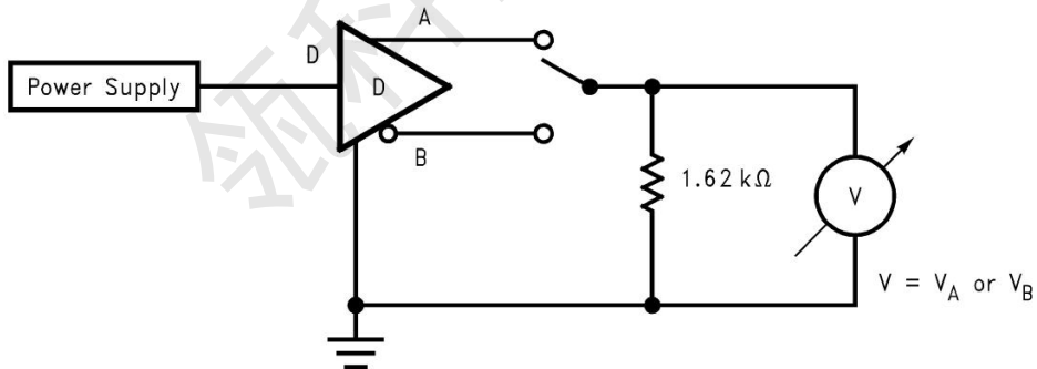
图 8 差分驱动 DC 开路测试电路
