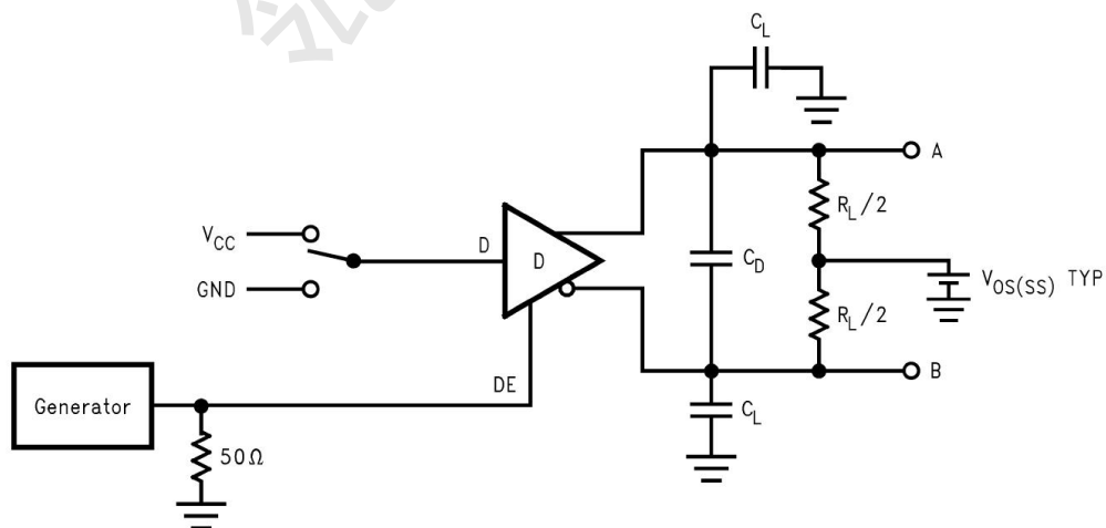
图 12 驱动器三态延时测试电路
