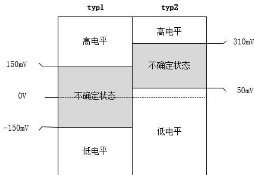
图 4 接收器模式示意图
