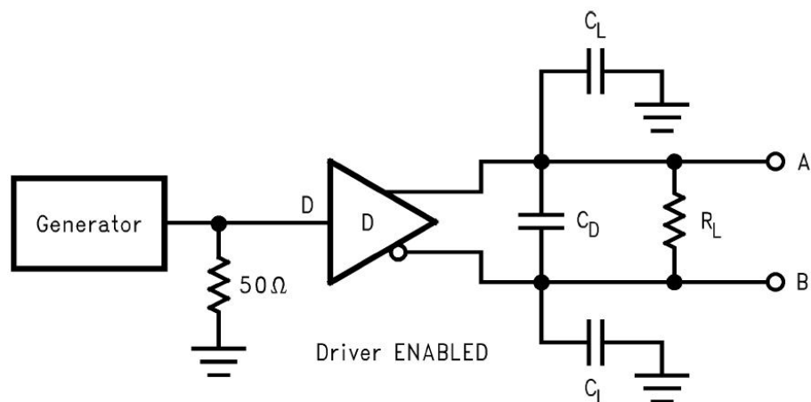
图 10 驱动器传输延时和传输时间测试电路
