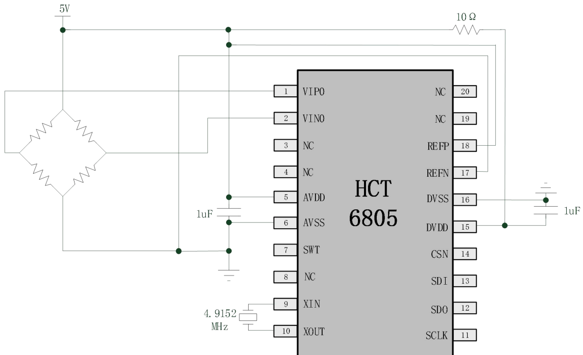
Figure 8-1 HCT6805 应用图 1
