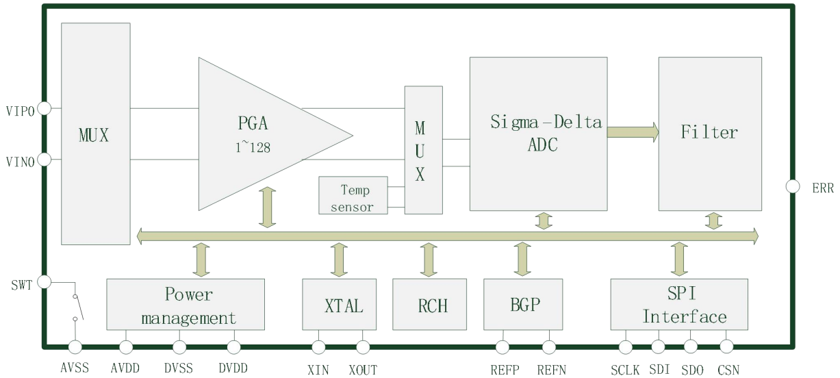
Figure 3-1 HCT6805 模块功能图
