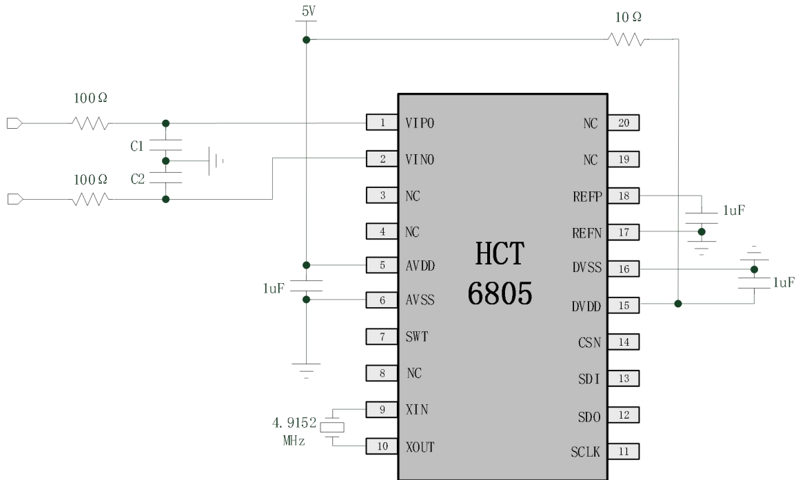
Figure 8-2 HCT6805 应用图 2
